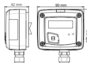
Modèle contact tuyauterie
