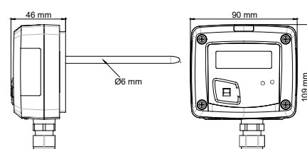
Modèle arrière inox*
